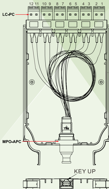
Item # UVR-F-GMPO/APC-MD4SM-Z
