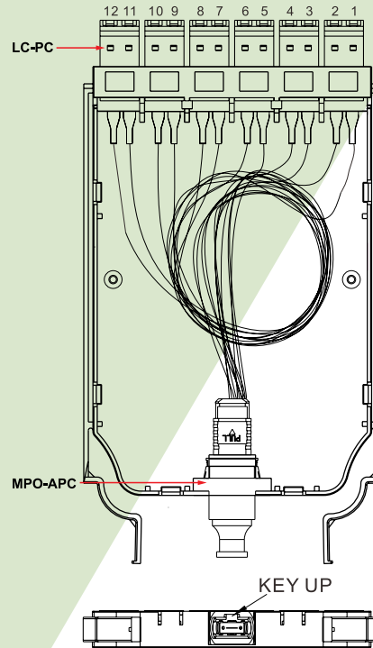
Item # UVR-F-GMPO-MD4OM4-Z
