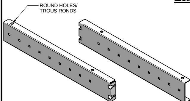
ITEM 1 INNER BRACKET FPRK2839 QTY 4
