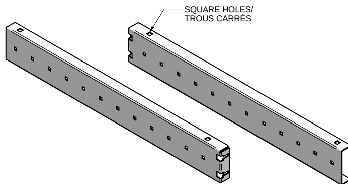
ITEM 1 INNER BRACKET FPRK3648 QTY 4
