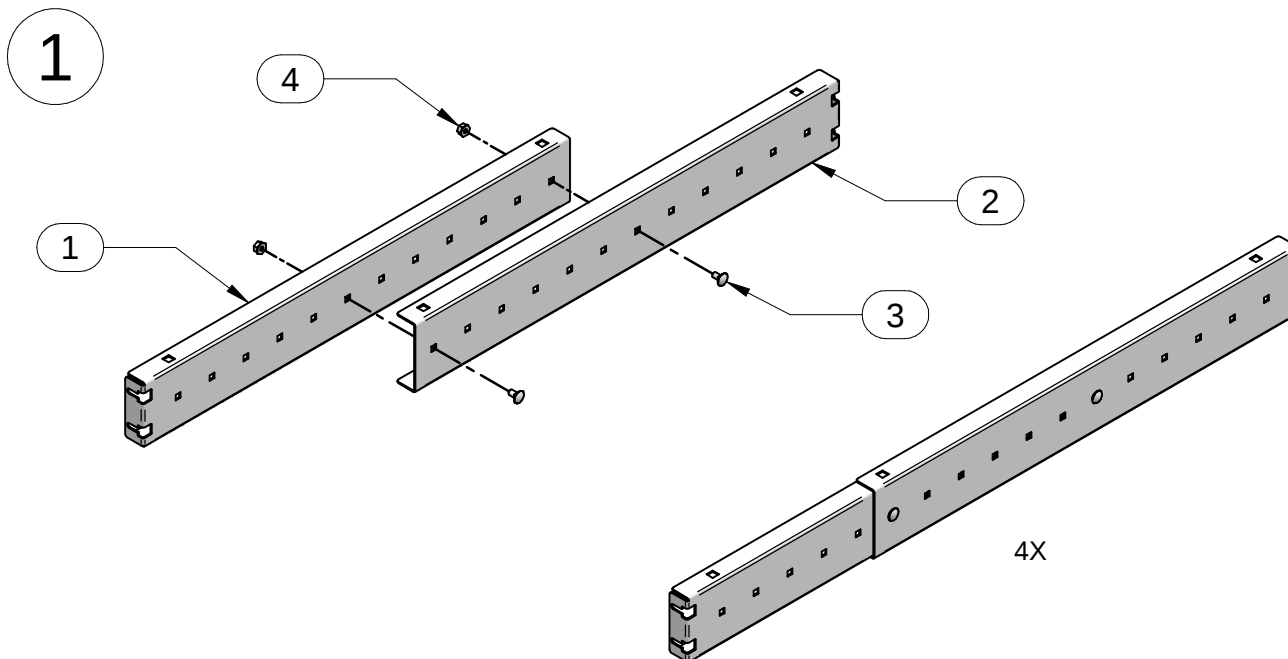
ITEM 3 1/4-20 x 1/2 CARRAGE BOLT QTY 8
