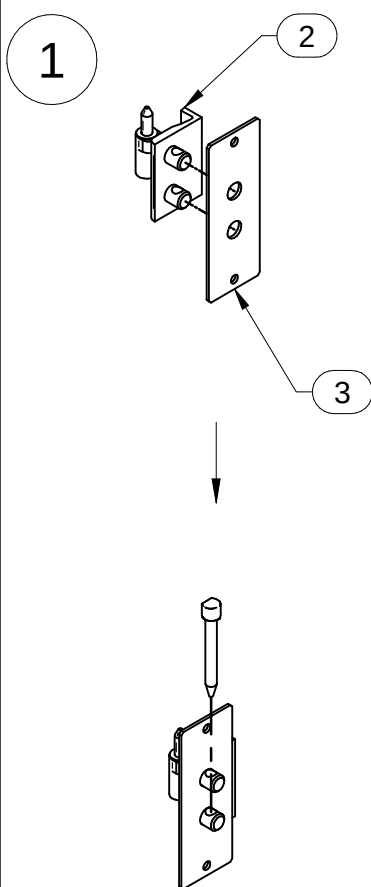
ITEM 1 RCK DOOR QTY: 1
